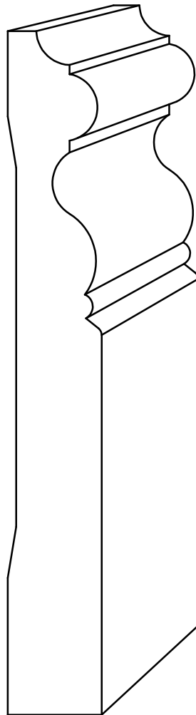
B 68 1 1/16" x 5" **
