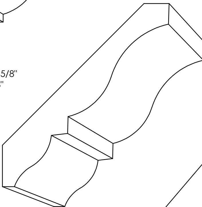
CR 3645 - 11/16'' \times 4-1/2'' P= 3'' - D= 3-3/8''
