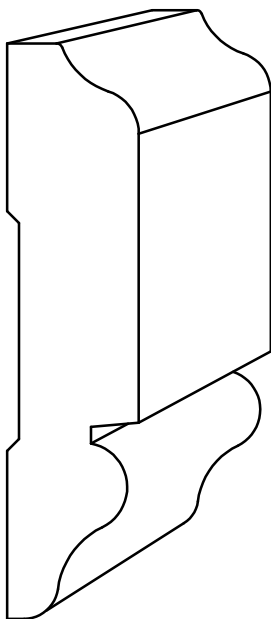
CHR 34 - 11/16" x 3"
