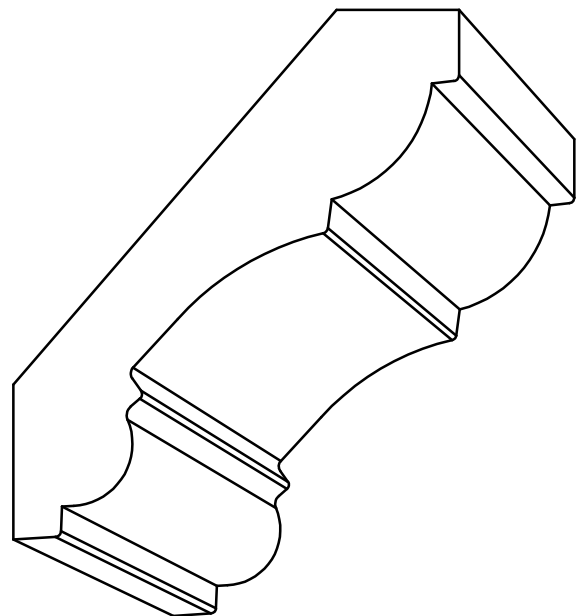
CR 3608 - \frac{3}{4}'' \times 3\frac{5}{8}'' P= 2\frac{5}{16}'' - D= 2\frac{3}{4}''
