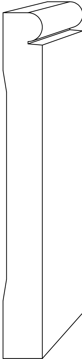
B 25 11/16" x 6" **
